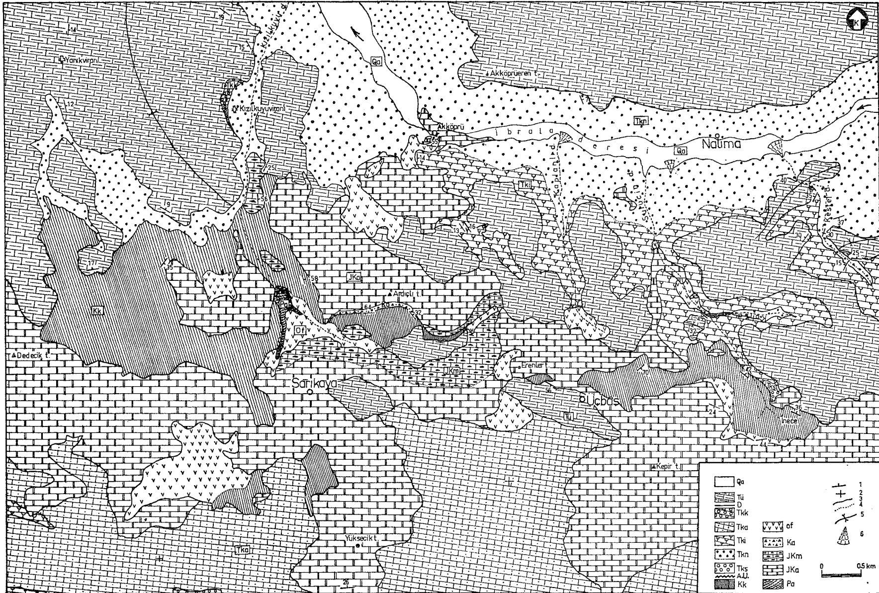
Sekil 2: Sarıkaya-Üçbaşı (Karaman) yöresinin jeoloji haritası. Qa-Alüvyon, Tü-Killi Kireçtaşı (Pliosen), D-Aeşiz uyumsuzluk, Tkk-Çakıltası (Helvesiyen), Tka-Kumlu kireçtaşı (Helvesiyen), Tki-Besif kireçtaşı (Helvesiyen), Tkn-Marn, Kumtaşı, çakıltası, kireçtaşı (Helvesiyen), Tks-Çakıltası (Helvesiyen), A.U.-Acılı uyumsuzluk, Kk-Badyolarit (Maestrihtiyen), Of-Ofiyolitli melanj, Ka-Bres (Maestrihtiyen), JKm-Çörtlü kireçtaşı (Malm-Apsiyen), JKa-Katmanlanmasız kireçtaşı (Malm-Apsiyen), Pa-Şist (Devonyen). 1 - Eğim ve doğrultu, 2 - Yatay katman, 3 - Dokanak, 5 - Olasılı dokanak, 5 - Senklinal, 6 - Alüvyon konisi.
